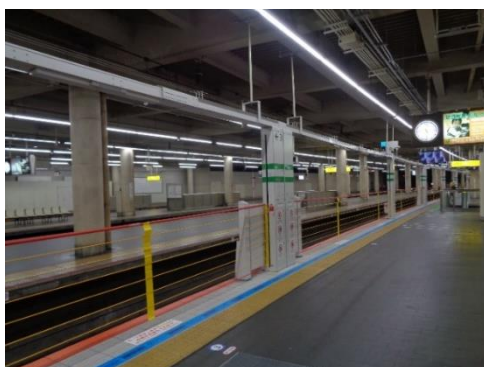
同型の昇降ロープ式ホームドア（大阪阿部野橋駅）
